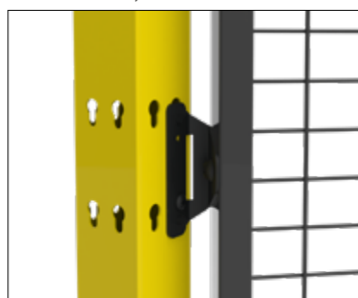
T01-01 O-fixation 180° Fixation avec un angle jusqu'à 180°. Cette fixation est utilisée lorsque la protection de machines doit être montée selon des angles autres que 90°.
