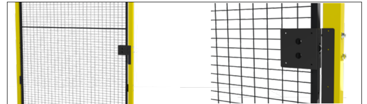
T10-32. Fixations, Schmersal AZM200 porte battante, droite/gauche.
