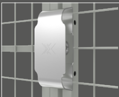
Hänglåsbeslag med heltäckande skyddskåpa (ingår som standard i FK) Kan användas på alla dörrar för att skydda hänglåset.
